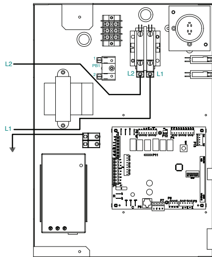
Figure 13B : Boîtier de commande pour tension de 208-230/60/1
