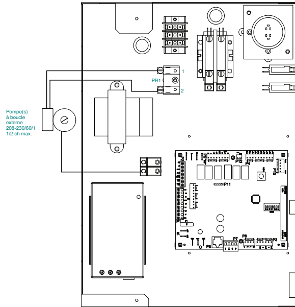
Figure 14 : Câblage de la pompe 208-230/60/1
