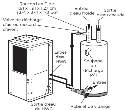
Figure 12 : Installation du générateur d'eau chaude dans le réservoir de préchauffage
