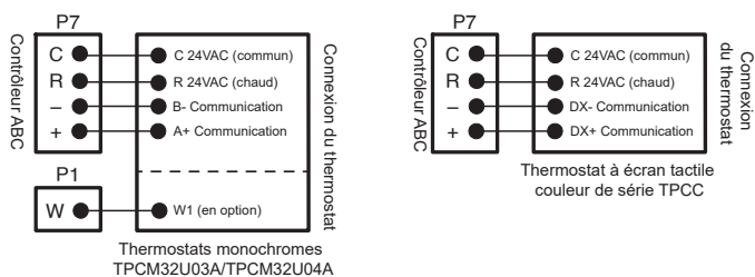
Figure 22 : Câblage du thermostat (signaux de communication)
